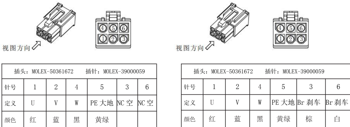
图 1 750W 以下电机动力线-不带刹车
